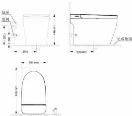
安装图
